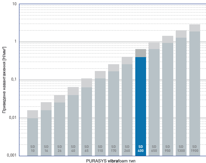
PURASYS vibrafoam типи Робочий інтервал навантажень
