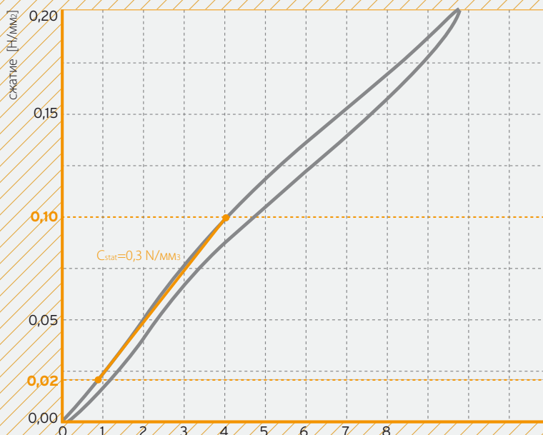
Кривая упругости подбалластного мата Sylodyn® DN 335
