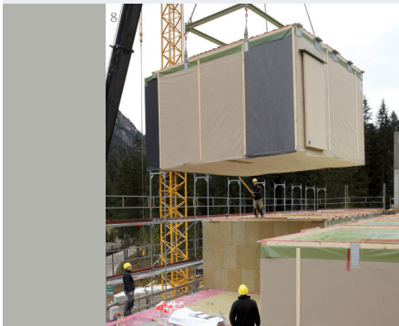
Модульная конструкция
