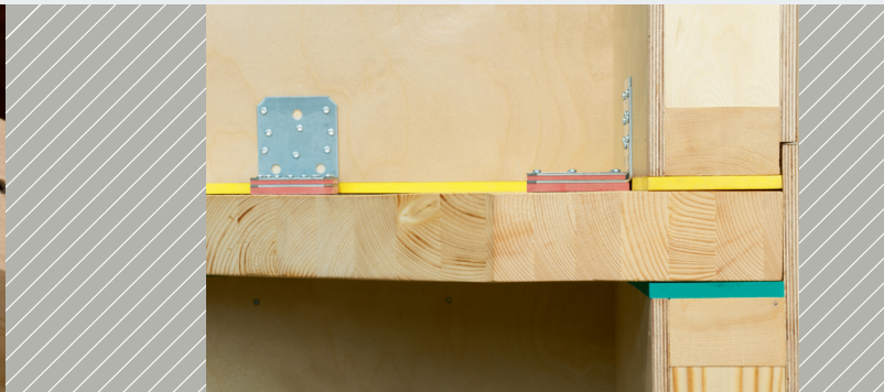
Упругая опора стены и перекрытия
