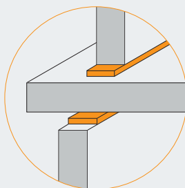
Установка на упругие опоры боковых элемен- тов конструкций
